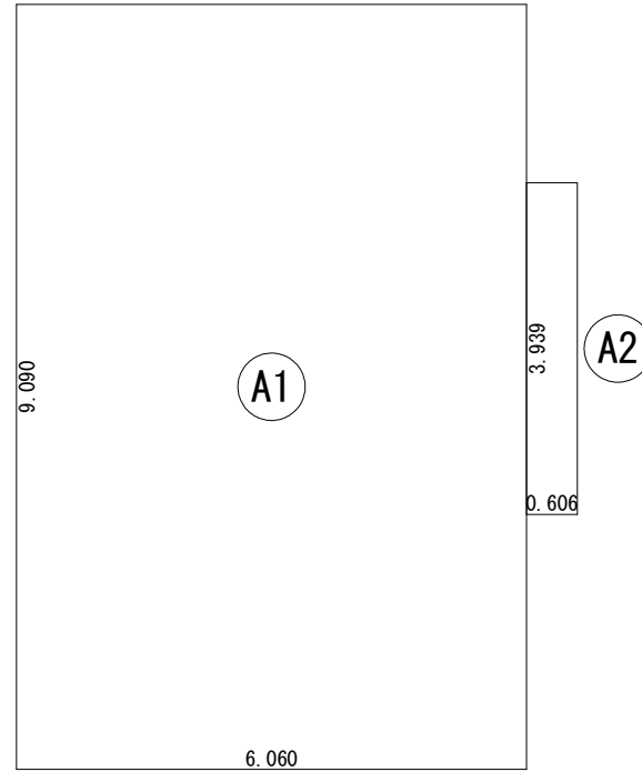
2階 床面積求積図 S:1/100
